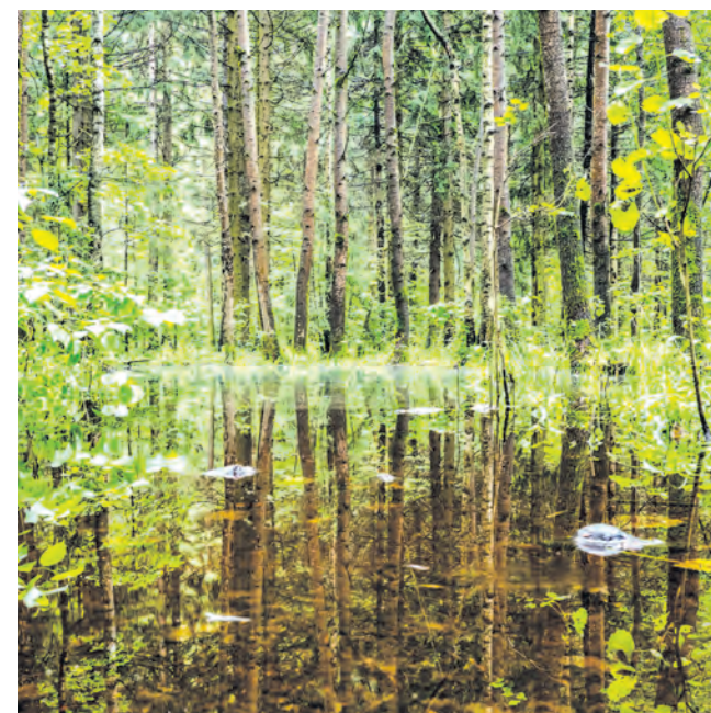
Малинское болото
